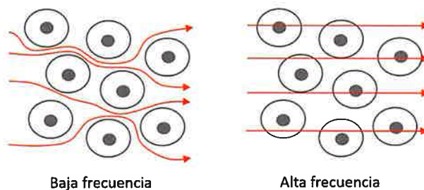
Figura 2. Flujo de corriente eléctrica a través de un medio biológico a baja y alta frecuencia.
