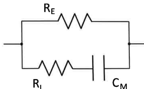
Figura 3. Modelo eléctrico simple de la bioimpedancia de un medio biológico.
